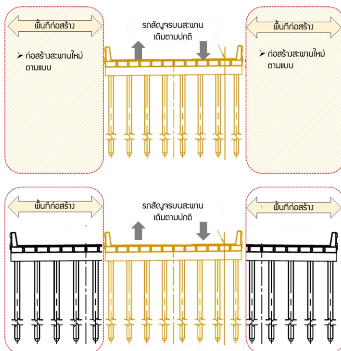
รูปที่ 6-12 การจัดการจราจรระหว่างก่อสร้างสะพาน ระยะที่ 1
