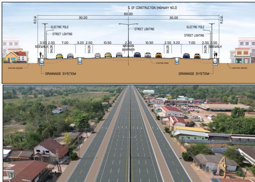
รูปที่ 5-1 รูปแบบทางหลวงหมายเลข 2 บริเวณย่านชุมชน
