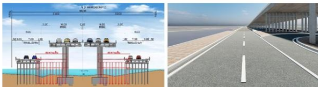
รูปที่ 5-3 ตำแหน่งและรูปแบบจุดกลับรถในโครงการ
