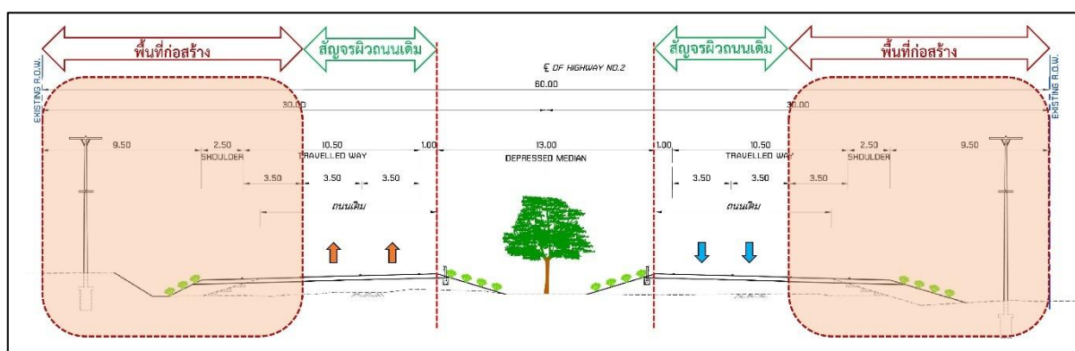
รูปที่ 6-2 การจัดการจราจรสำหรับการก่อสร้างสะพานข้ามทางแยก ระยะที่ 1
