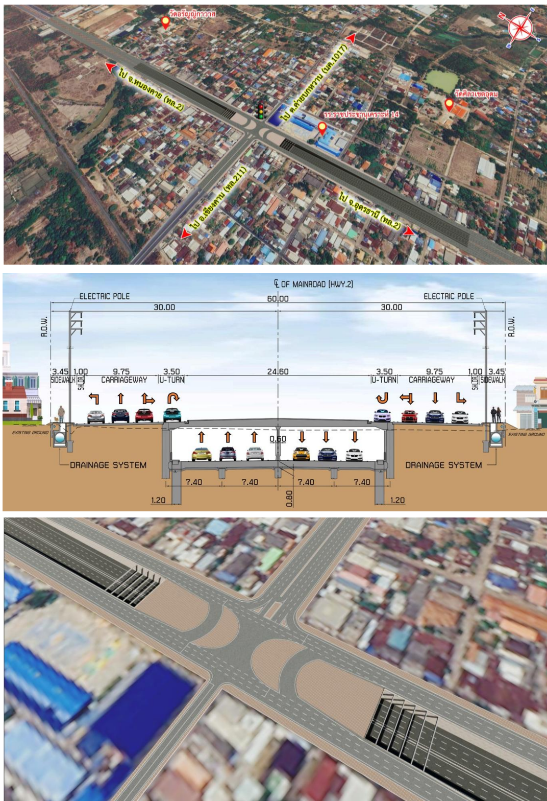
รูปที่ 5-6 รูปแบบทางแยกต่างระดับบริเวณทางแยกหนองสองห้อง
